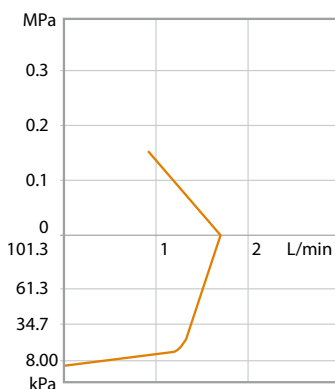
MDG-M2B□24
