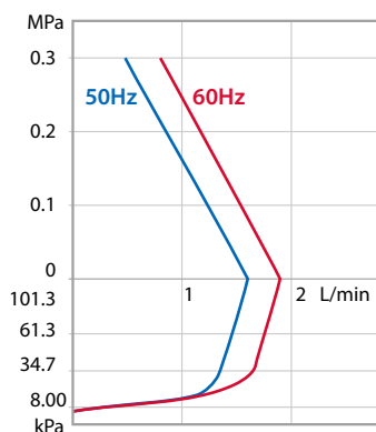
MDG-R2B□B230
