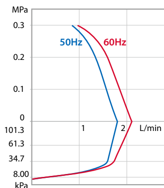
MDG-R2R□B230
